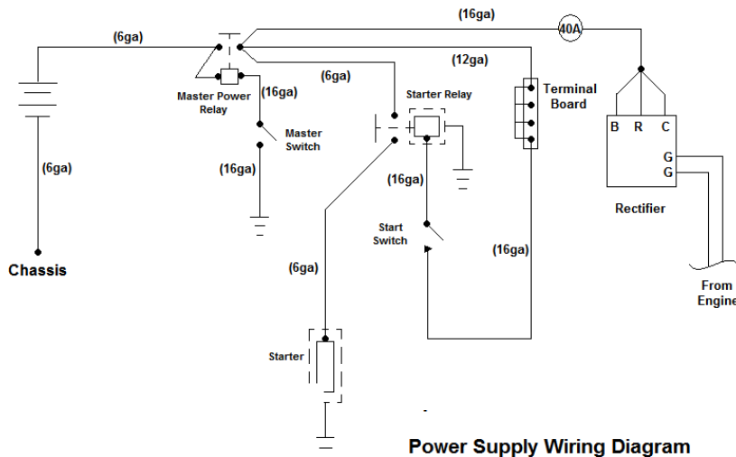
REVO Rotax 912 UL & 912 ULS Wiring
